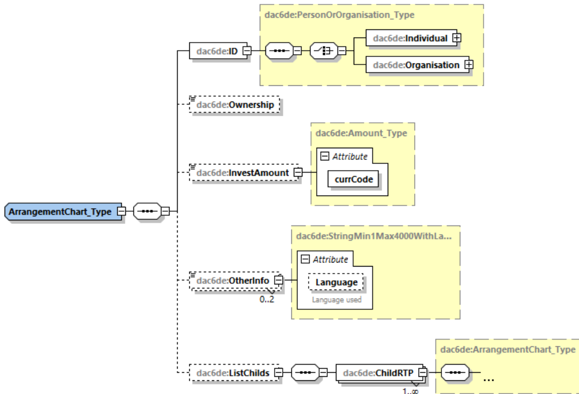
Abbildung 3: XML-Struktur ArrangementChart_Type
