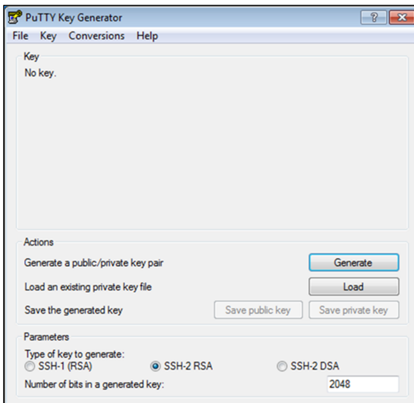
Abbildung 22: Key Generator Startseite
